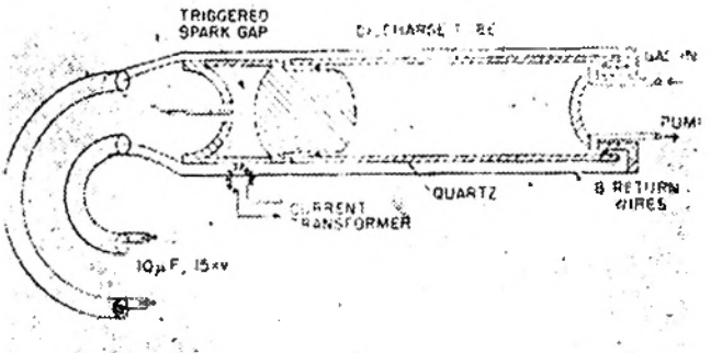
Desenho esquemático do cilindro magnetizado vendo-se os circuitos electricos usados para "empurrar" os gases aquecidos no centro do cilindro para deixar as paredes do mesmo frias. Nenhum material conhecido poderia suportar a temperatura de 100 milhões de graus Fahrenheit necessaria ao processo de fusão.
