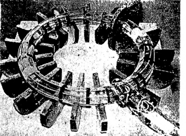
Os primeiros aparelhos de pesquisas de fusão controlada foram tubos de vidro circulares com fios de arame do lado externo. Quando terminado, o aparelho se parecia com o da foto. Um imã de seis toneladas foi usado para conseguir as linhas magneticas de força para confinar os gases superaquecidos no centro do tubo.
